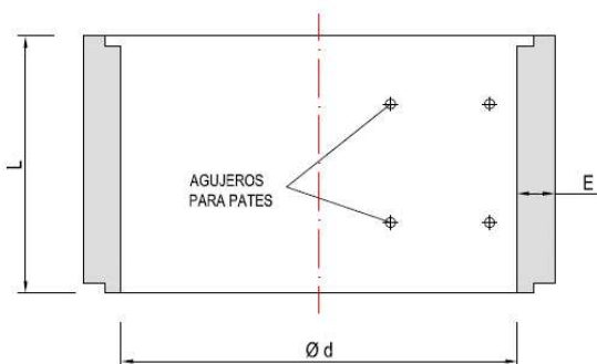
SECCION TIPO
